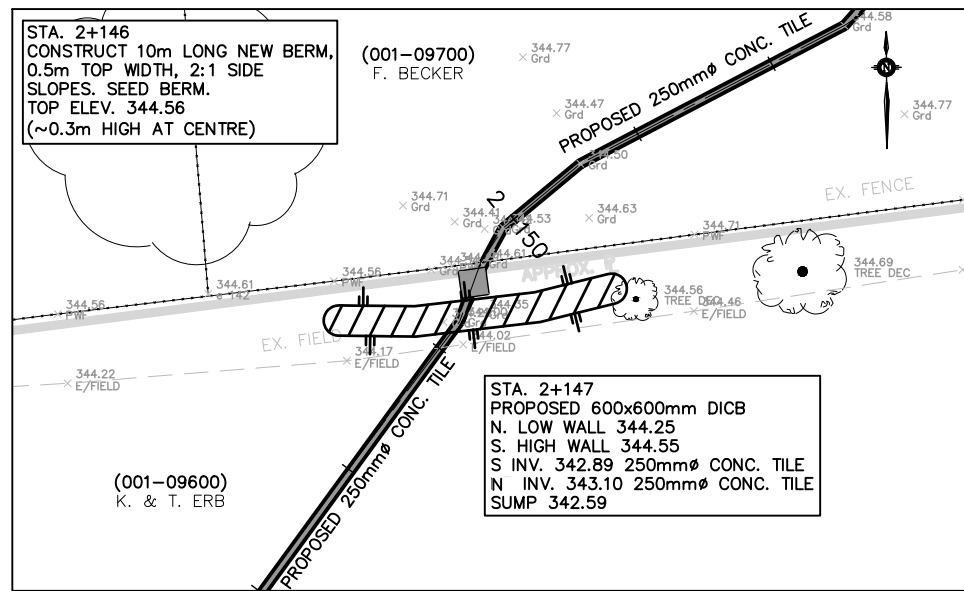
STA. 2+147: DETAIL
