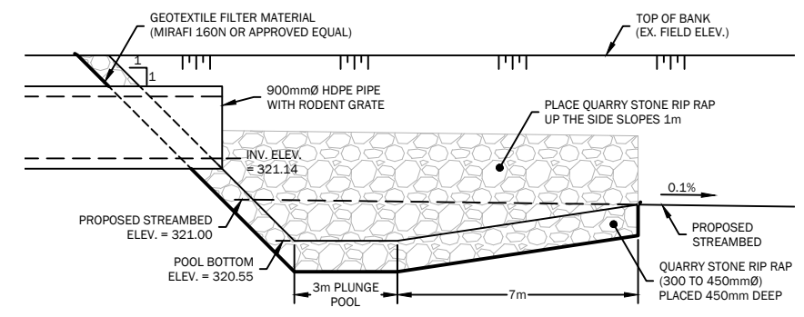
PLUNGE POOL DETAIL N.T.S.
